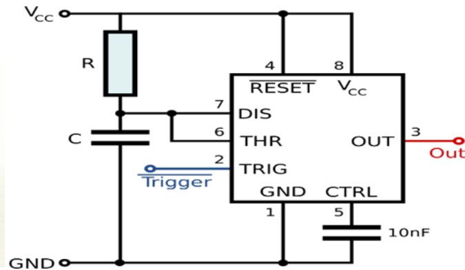
Fig.25- 555 IC Timer layout
