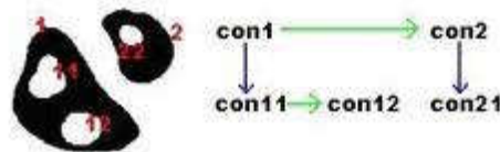
OpenCV 轮廓检测 CV_RETR_TREE 参数示意图
